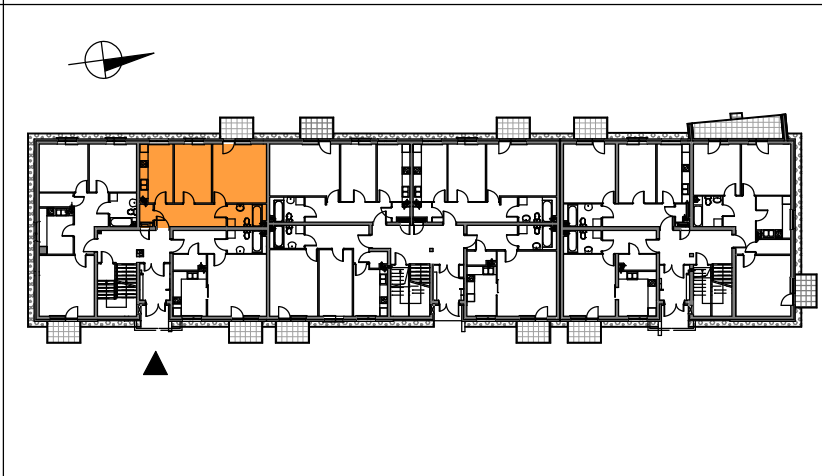
SCHEMAT ROZMIESZCZENIA MIESZKAŃ BUDYNKU NR 2
