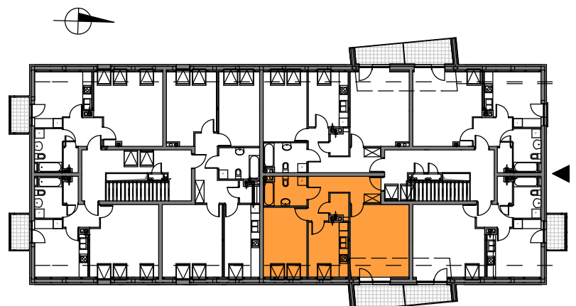
SCHEMAT ROZMIESZCZENIA MIESZKAŃ BUDYNKU NR 7
