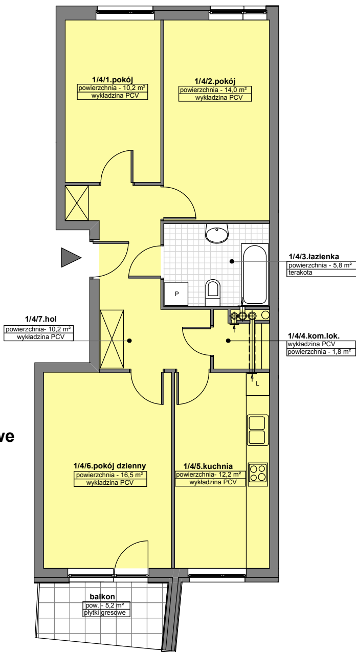
SCHEMAT ROZMIESZCZENIA MIESZKAŃ BUDYNKU NR 7
