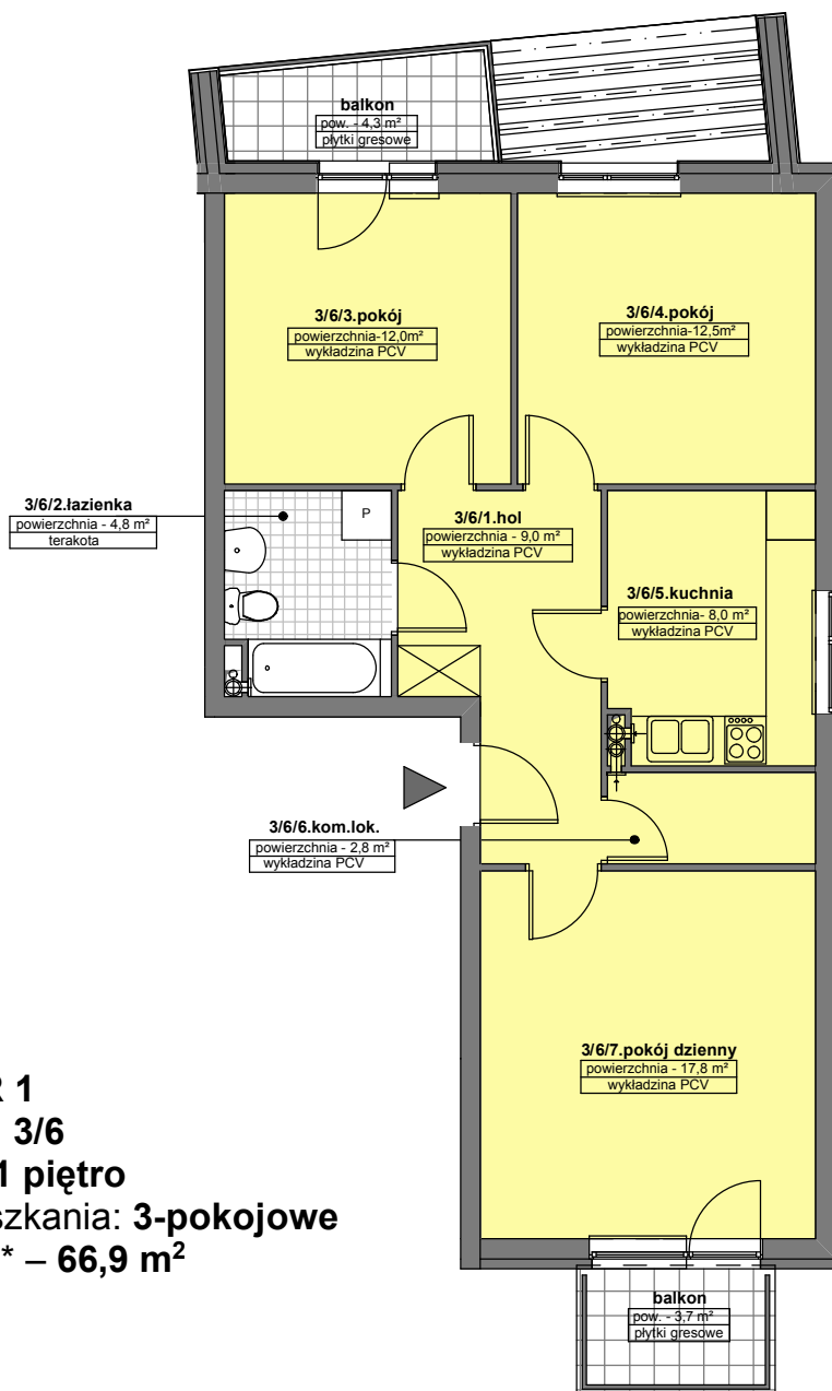
SCHEMAT ROZMIESZCZENIA MIESZKAŃ BUDYNKU NR 1
